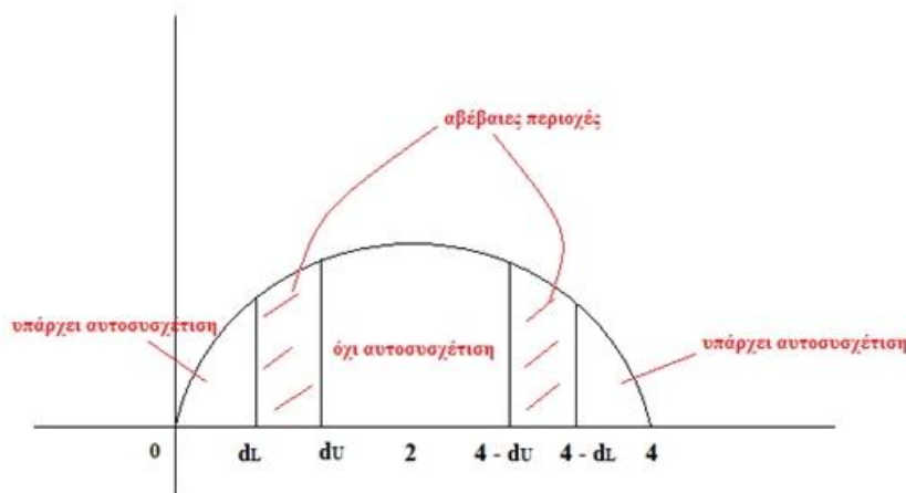
Διάγραμμα 6: Durbin-Watson stat
